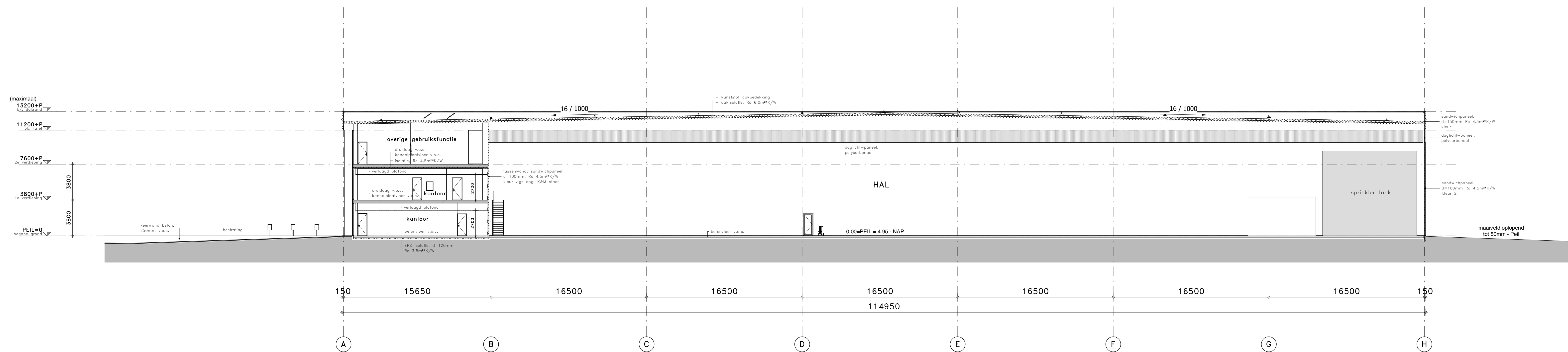
DOORSNEDE A-A
